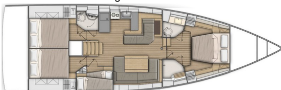
Versione 4 cabine 4 locali bagno:
